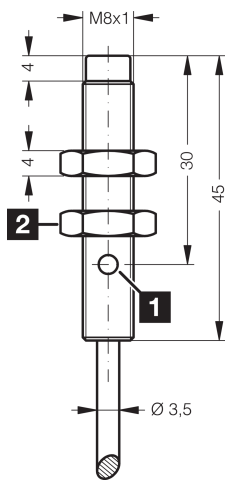
1) LED 2) Schlüsselweite 13 mm BK: schwarz BN: braun BU: blau
