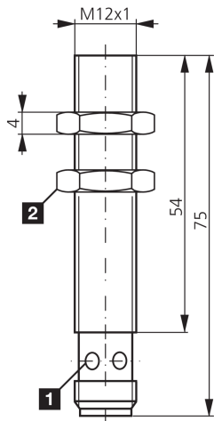
2) Schlüsselweite 17 mm
