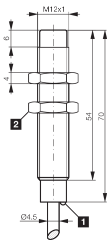
2) Schlüsselweite 17 mm
