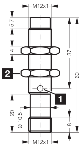
1) LED 2) Schlüsselweite 17 mm BK: schwarz BN: braun BU: blau
